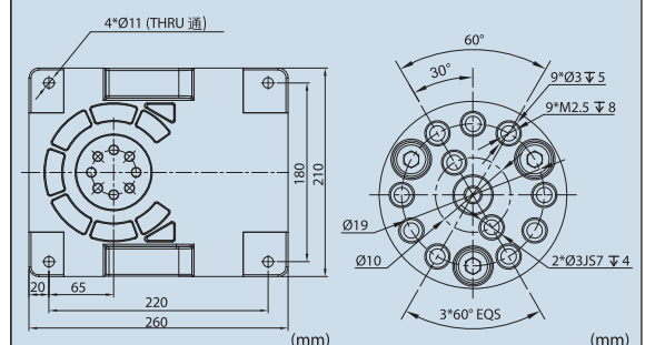
Base Mounting Face 底板安装尺寸
